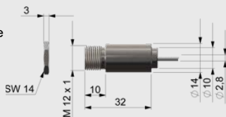
Messkopf (eingebaute CF-Linse)
