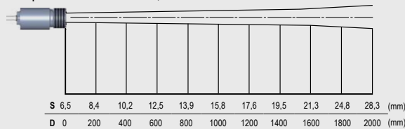
Optik CT 3MH1-H4 SF, D:S = 75:1
