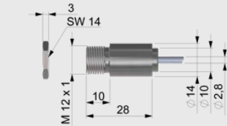
Messkopf
