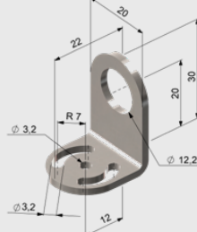
Montagewinkel, fest (ACCTFB)
