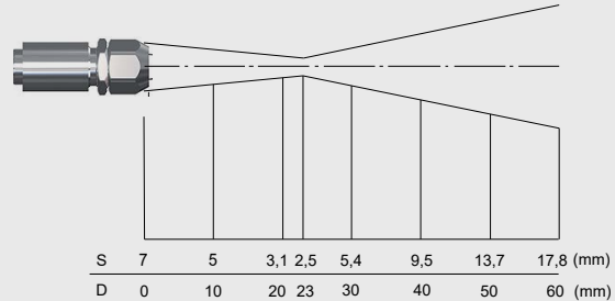
Optik mit CF-Vorsatzlinse, D:S = 2:1 (Fernfeld = 2,5:1)
