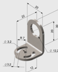
Montagewinkel, fest (ACCTFB)
