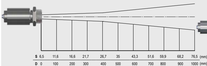
SF-Optik, D:S = 15:1
