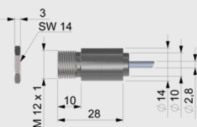
Abmessungen CSmicro
