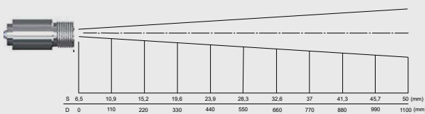
SF-Optik, D:S = 22:1
