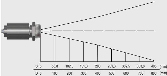
SF-Optik, D:S = 2:1
