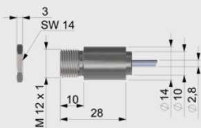
Abmessungen optris® CSmicro 3M CF1
