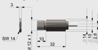
Abmessungen optris® CSmicro 3M CF1
