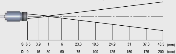
Optik CSmicro 3MH CF1, D:S = 33:1 (Fernfeld 4:1)
