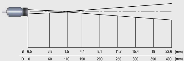
Optik CF, D:S = 75:1
