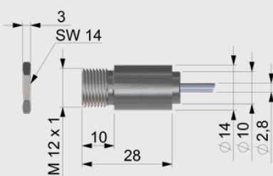
Abmessungen CSmicro
