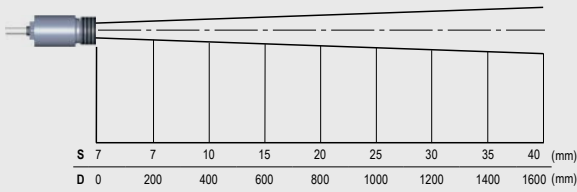
Optik SF, D:S = 40:1
