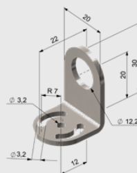
Montagewinkel, fest (ACCTFB)
