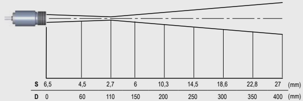
Optik CF, D:S = 40:1
