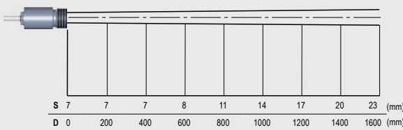
Optik SF, D:S = 75:1
